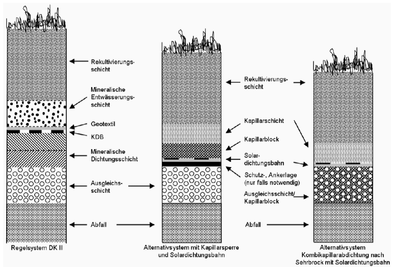
Abb. 3: Integration der innovativen Photovoltaikanlage als Abdichtungselement in zwei Varianten einer alternativen Kombinationsabdichtung für ein Klasse 2 Deponie im Vergleich zum Regelsystem nach TA-Siedlungsabfall
