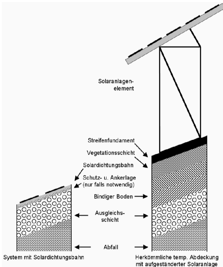
Abb. 2 Temporäre Deponieabdichtung in Kombination mit einer Photovoltaikanlage als innovatives und zum Vergleich als konventionelles System
